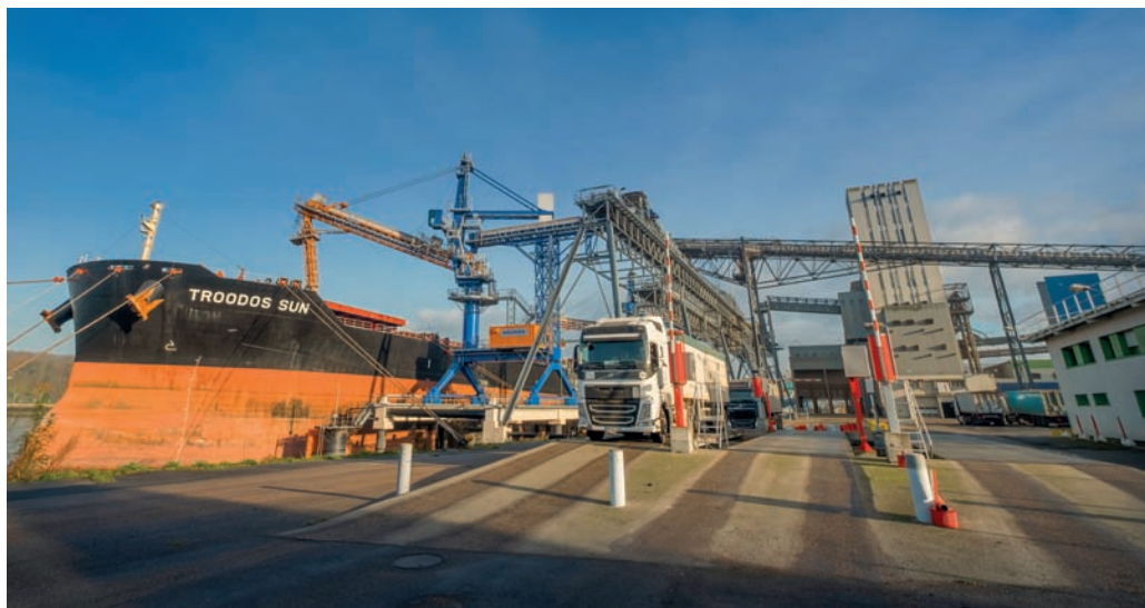
Chargement d'un navire sur le site Sénalia de Grand-Couronne avec les nouveaux portiques, qui permettent de charger à 3000 t/h sans émanation de poussière.
